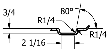
SECTION B-B SCALE 0.125 : 1
