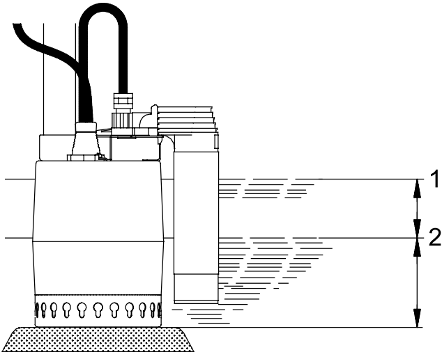
Start/stop levels for UNILIFT KP AV
