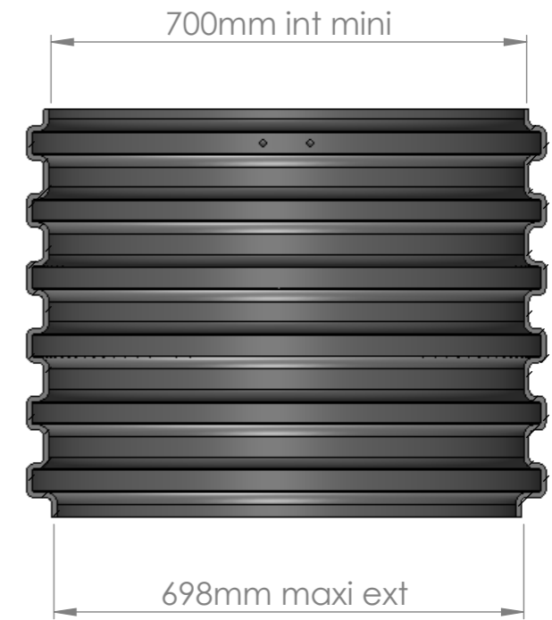
COUPE B-B
