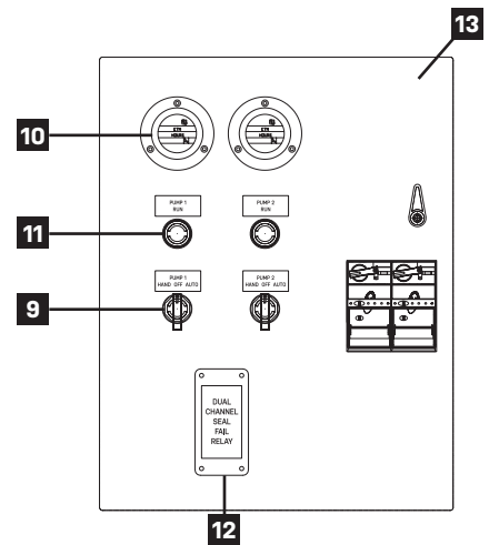
Inner Door
